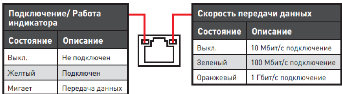
Рисунок 5 – Состояния индикаторов соединителей RJ-45
