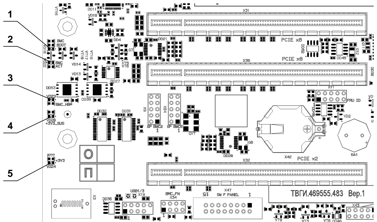
Рисунок 6 - Расположение светодиодов на панели 1Э8СВ-иАТХ
